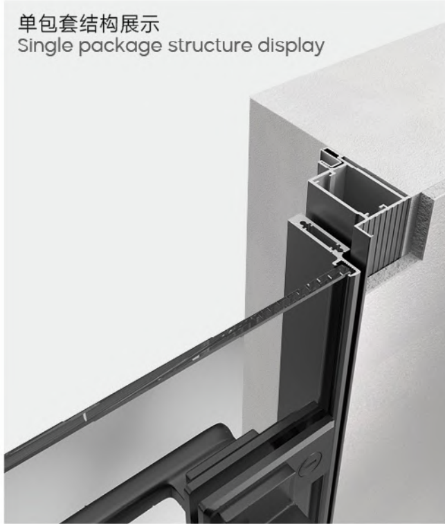
双隐包套结构展示 Double hidden package structure display
