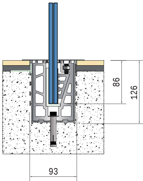
尺寸 Detail
