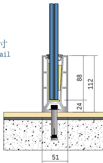
DK01 亚克力板 Acrylic
