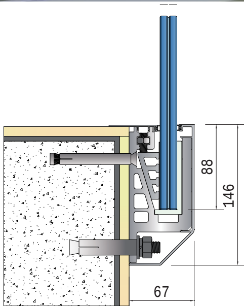
尺寸 Detail
