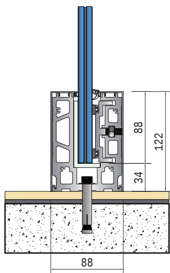
尺寸 Detail
