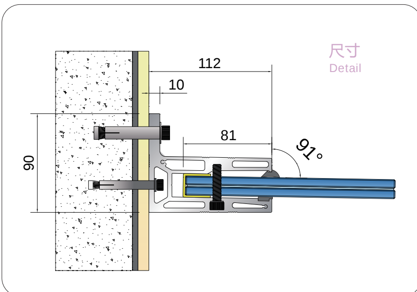
底座 Base Profile
