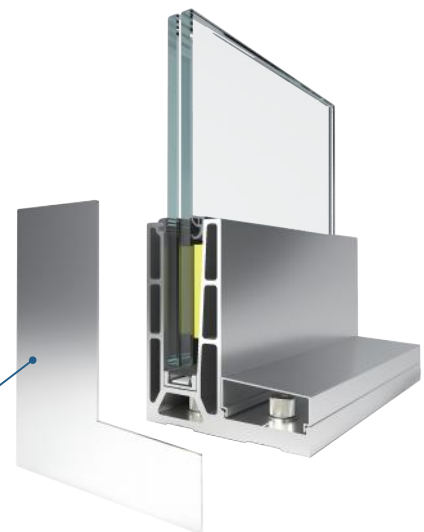
A3004 不锈钢板/铝板 SS/Alu Panel
