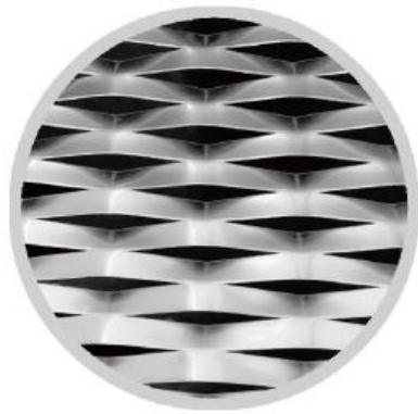
网 孔: 50*160MM 梗 宽: 22.5MM 开孔率: 10%
