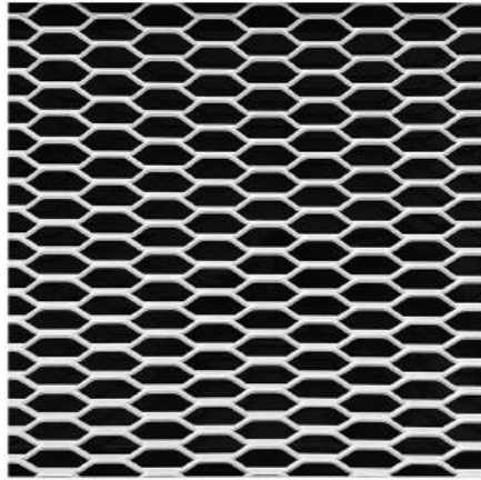
网 孔: 13*50mm 厚 度: 2.0mm 梗 宽: 2.5mm 开孔率: 61.5%
