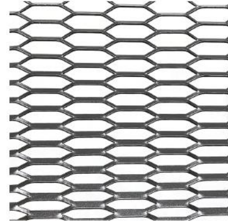
网 孔: 20*100mm 厚 度: 2.0mm 梗 宽: 5mm 开孔率: 50%
